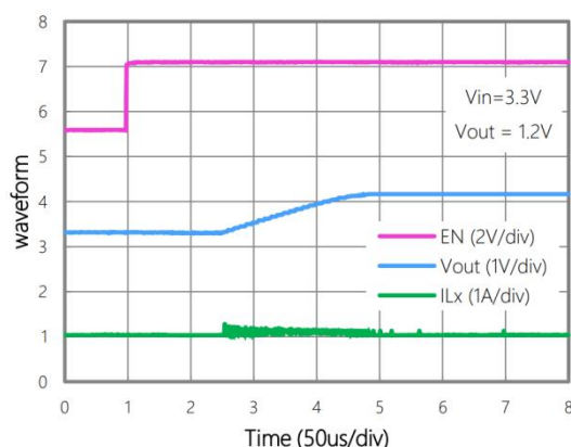
EN Startup
